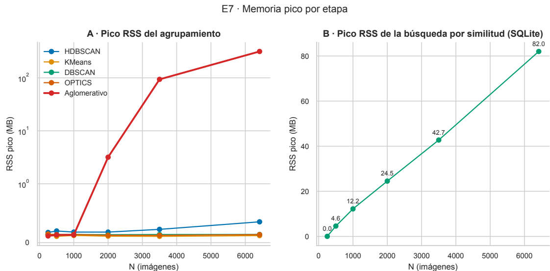
Figura 14: E7: memoria pico por etapa. El aglomerativo materializa la matriz O(n^2) de distancias y crece cuadráticamente con N ; HDBSCAN, DBSCAN y OPTICS se mantienen sublineales.
