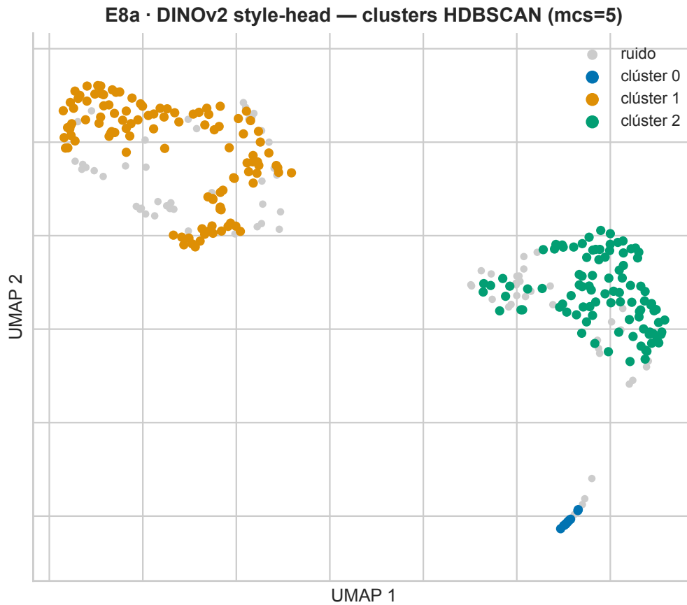
Figura 16: Representación bidimensional de la distribución de los recortes de E8a en el espacio de características de la cabeza estilística de DINOv2, coloreados por los tres clústeres generados por HDBSCAN.
