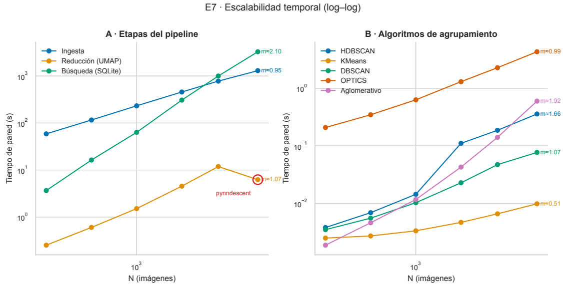
Figura 13: E7 (figura titular): tiempo de pared vs N por etapa del pipeline , escala log-log. La pendiente de la búsqueda por similitud SQLite ( \approx 2,10 ) confirma el coste O(n^2) por pasada. La caída de UMAP a N = 6416 refleja el cambio interno a pynndescent .
