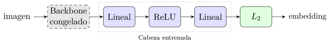
Figura 5: Cabeza de proyección ajustada a grafiti. El backbone permanece congelado y solo se entrena una secuencia ligera de capas para luego normalizar la salida a norma unitaria.
