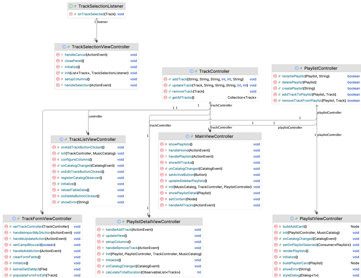
Figura 6: Diagramma delle classi — Controller e View (MVC)
