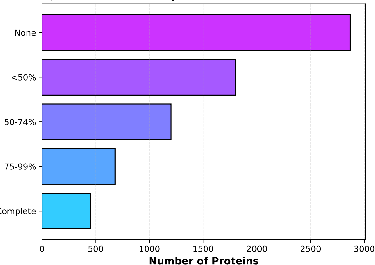
C) KEGG Module Completeness
