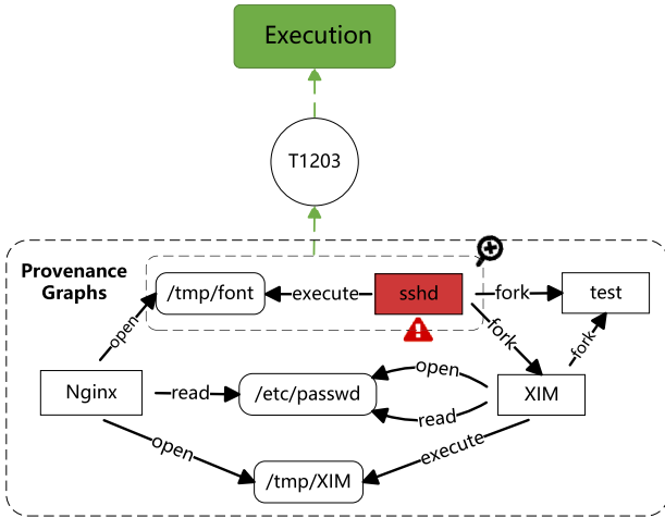
Fig. 4. An example of TTP matching from anomalous node behavior.
