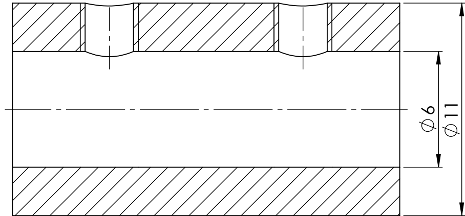
SECCIÓN C-C ESCALA 5 : 1
