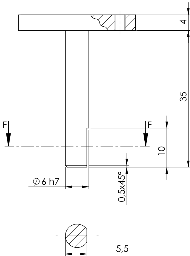
SECCIÓN F-F ESCALA 2 : 1
