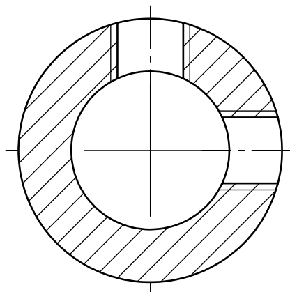
SECCIÓN C-C ESCALA 5 : 1
