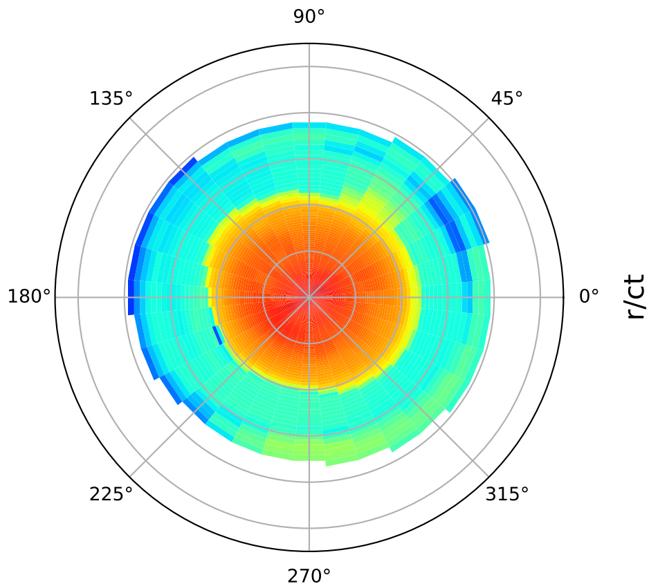
SFHo_q1.0 at t= 1000.05ms
