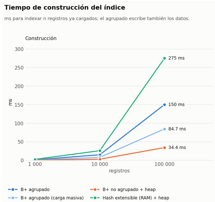
Figura 2: Tiempo de construcción del índice.
