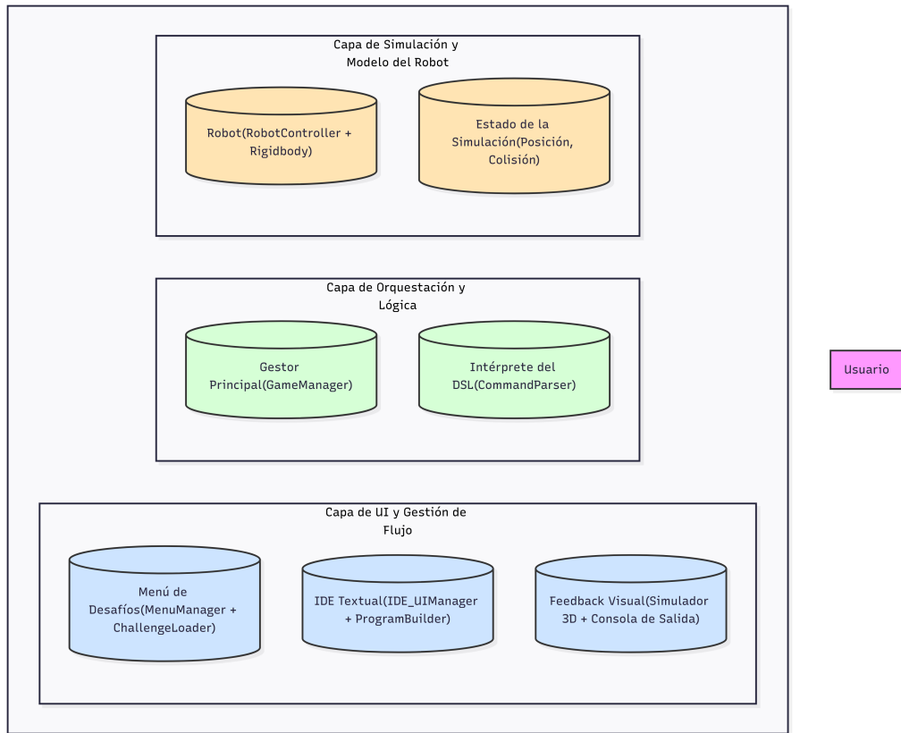
Figura C.5: Diagrama de componentes sistema DSL.
