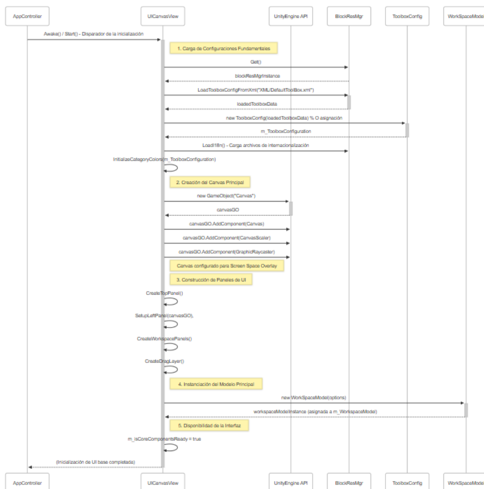
Figura C.6: Diagrama de secuencia: Inicialización interfaz principal.
