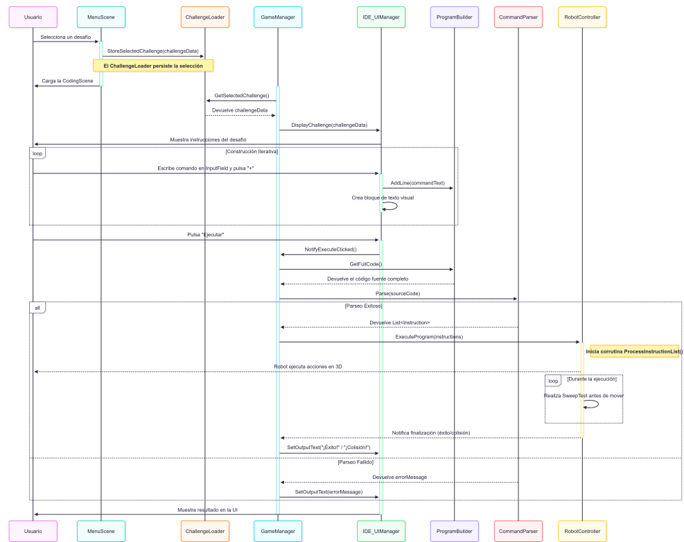
Figura C.13: Diagrama de secuencia: Flujo de ejecución del programa textual.
