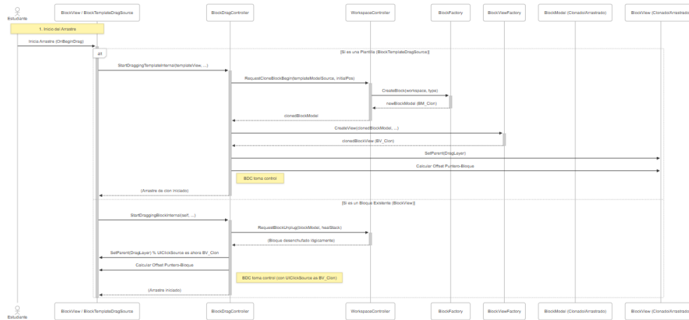
Figura C.8: Diagrama de Secuencia: Inicio del arrastre de un bloque.
