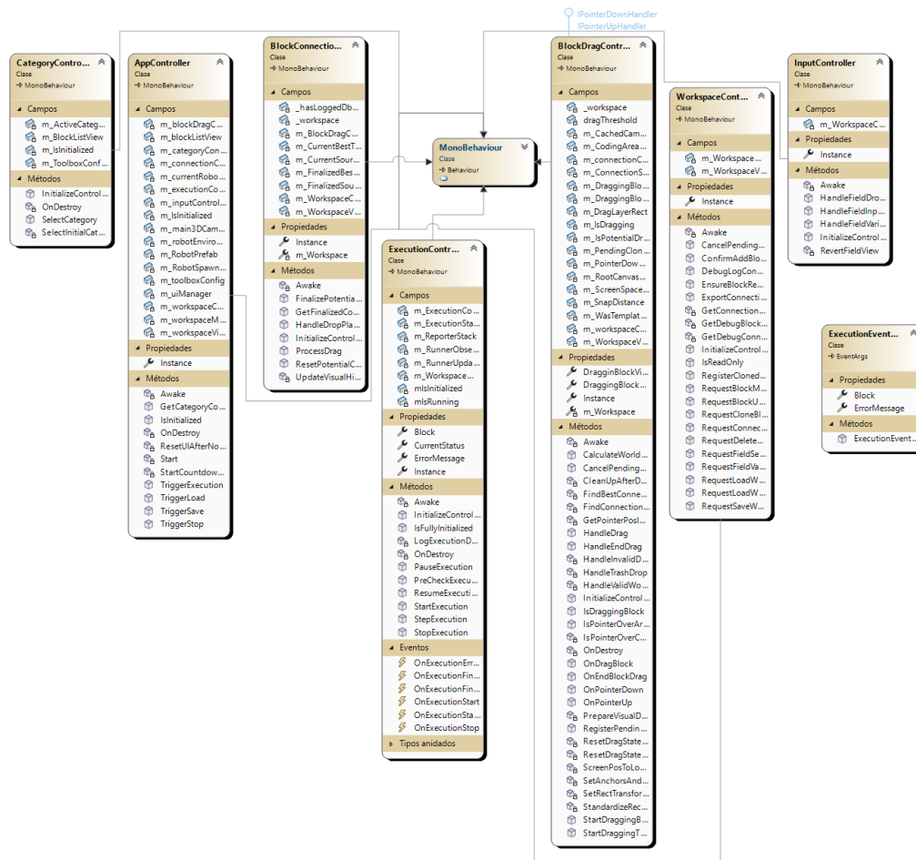
Figura C.4: Diagrama de clases de la capa controlador.
