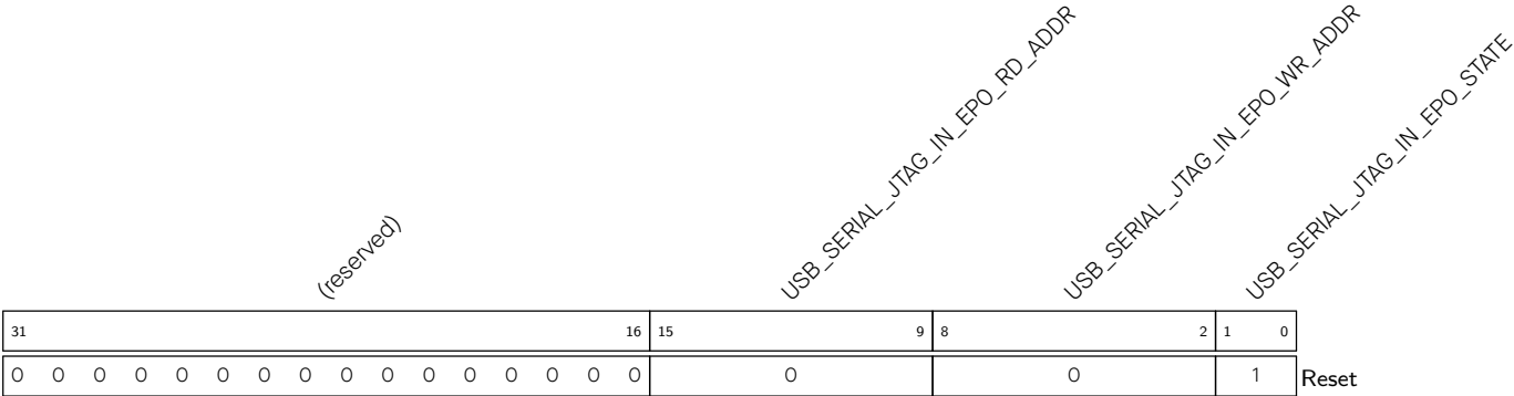
Register 33.13. USB_SERIAL_JTAG_IN_EPO_ST_REG (0x0028)
