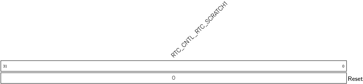
Register 10.19. RTC_CNTL_RTC_STORE1_REG (0x0054)
