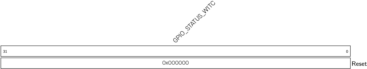
Register 6.29. GPIO_STATUS_W1TC_REG (0x004C)
