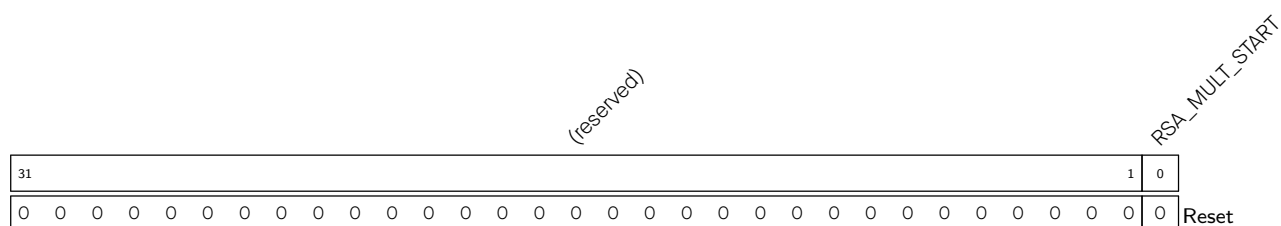
Register 20.6. RSA_MULT_START_REG (0x0814)
