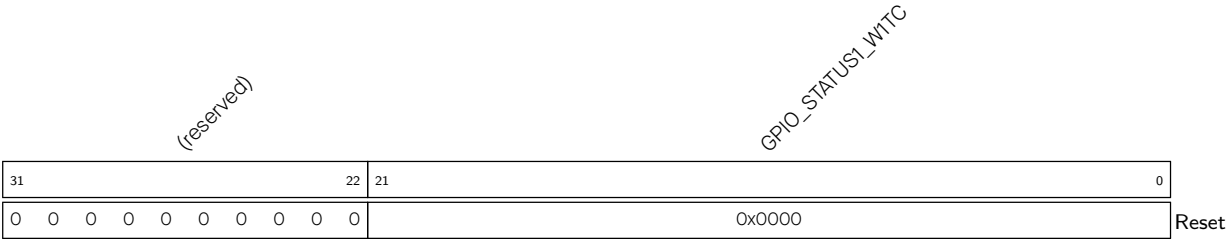
Register 6.31. GPIO_STATUS1_W1TC_REG (0x0058)
