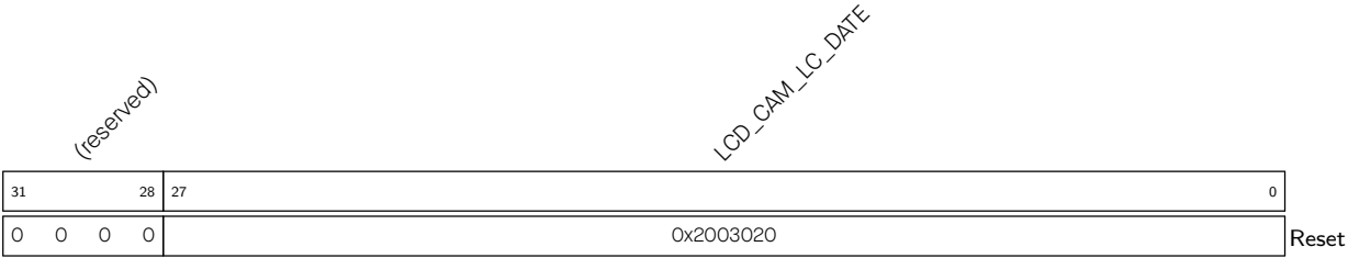
Register 29.18. LCD_CAM_LC_REG_DATE_REG (0x00FC)
