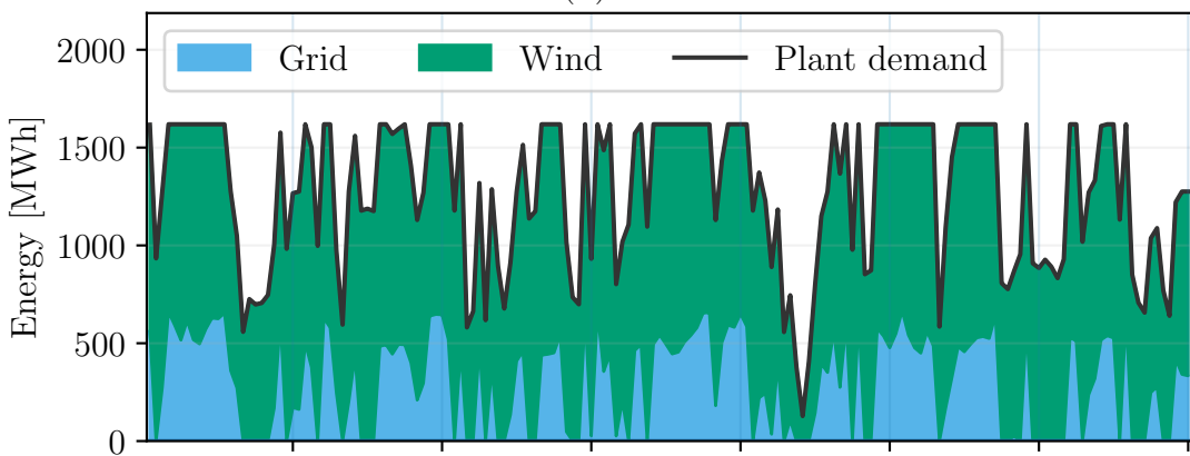
(b) Scenario 2
