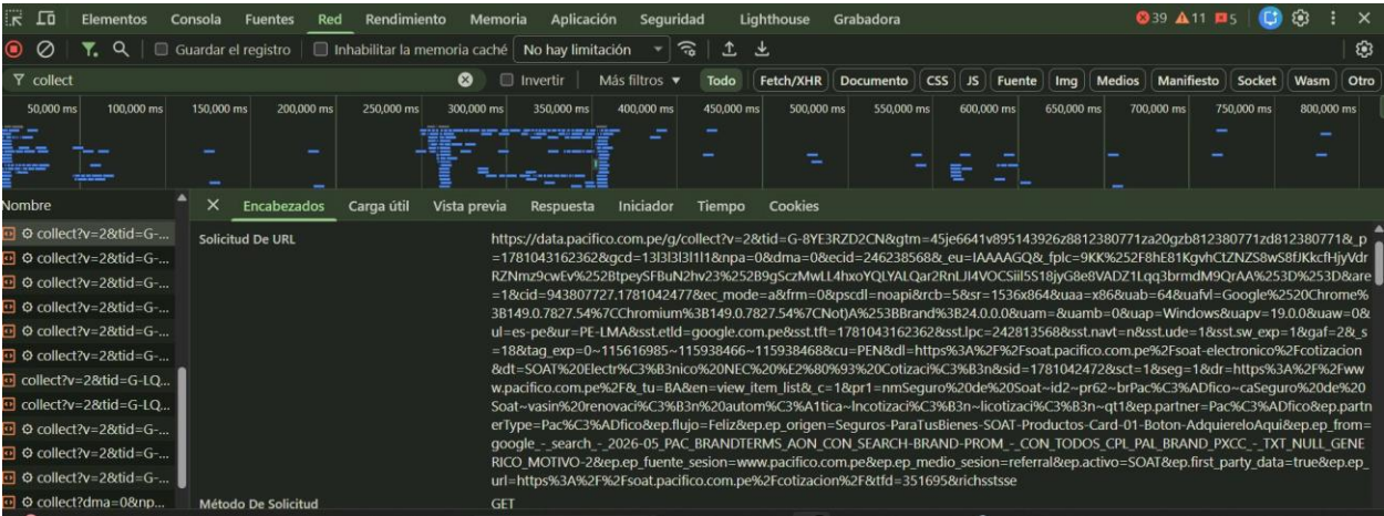
Figura 4 — Request al servidor proxy propio de Pacífico (data.pacifico.com.pe/g/collect), evidencia del Server-Side Tagging
