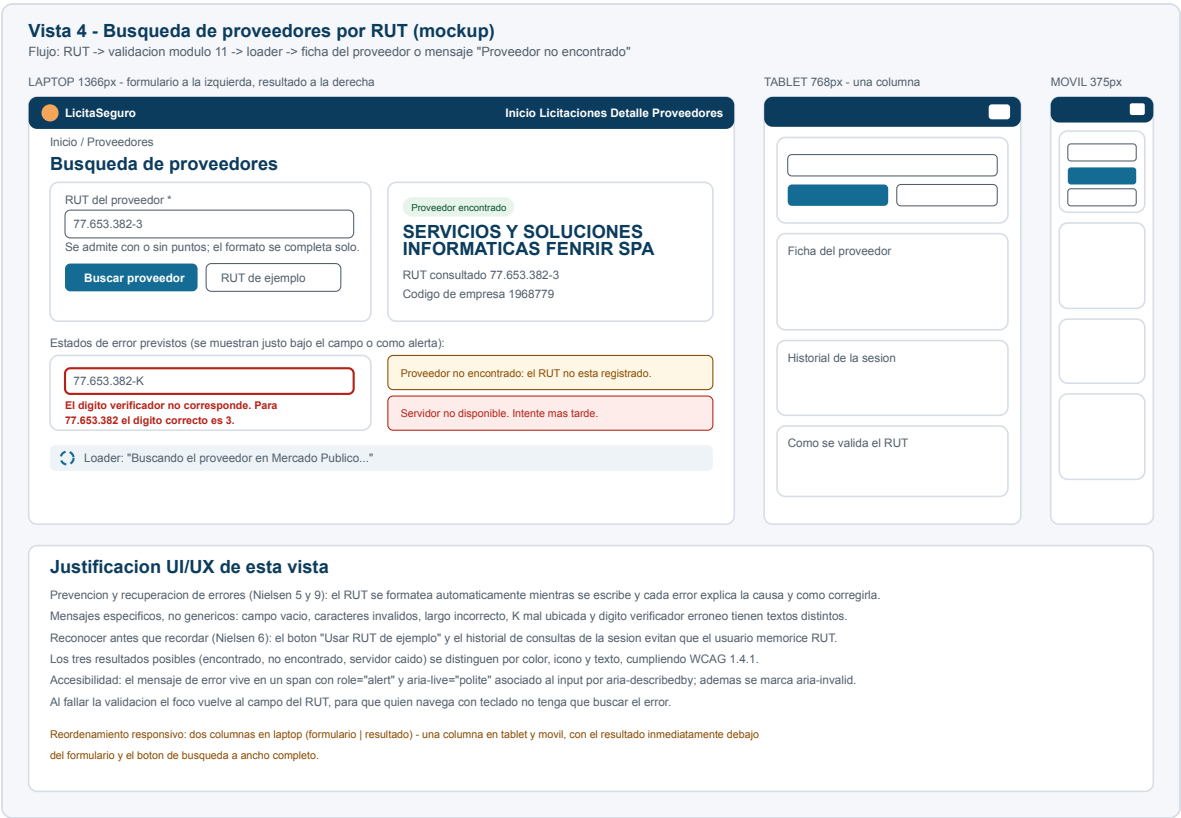
Figura 4. Mockup de la Vista 4 (busqueda de proveedores y estados de error).
