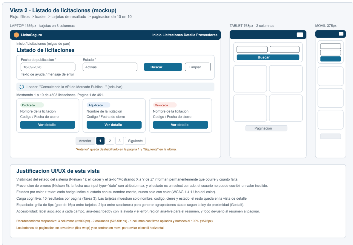
Figura 2. Mockup de la Vista 2 (listado con filtros, loader y paginacion).
