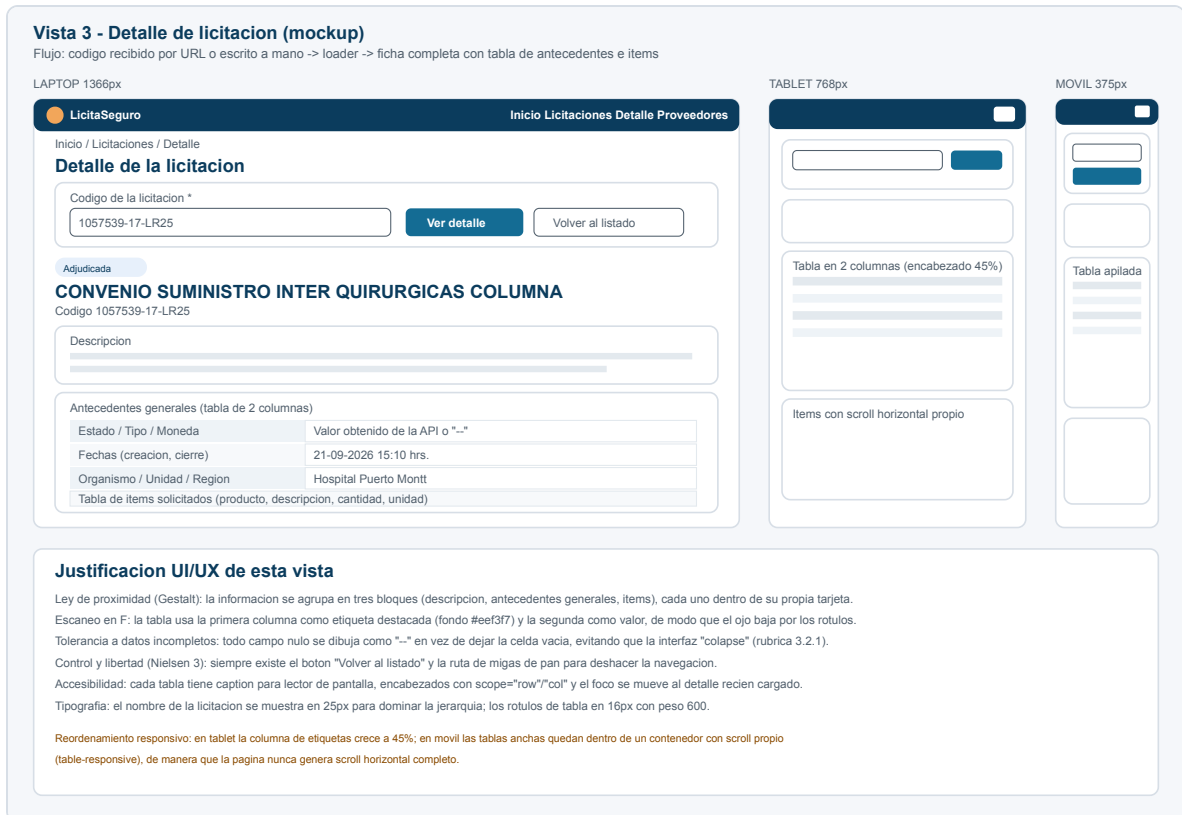
Figura 3. Mockup de la Vista 3 (detalle de licitacion).
