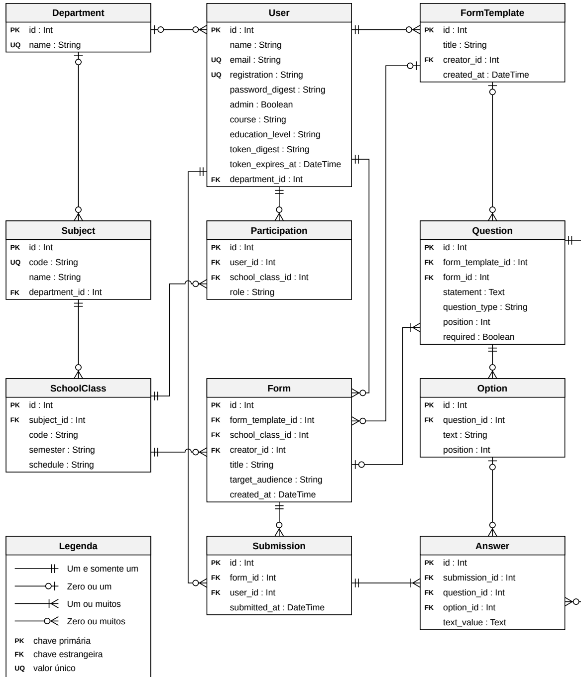
Figura 1: Modelo Relacional UML da aplicação CAMAAR.
