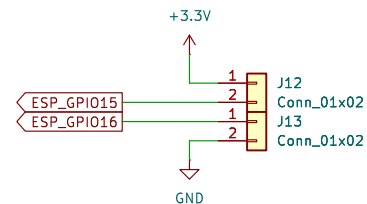
Encoder Motor 3
