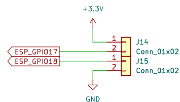
Encoder Motor 4
