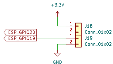
Encoder Motor 1
