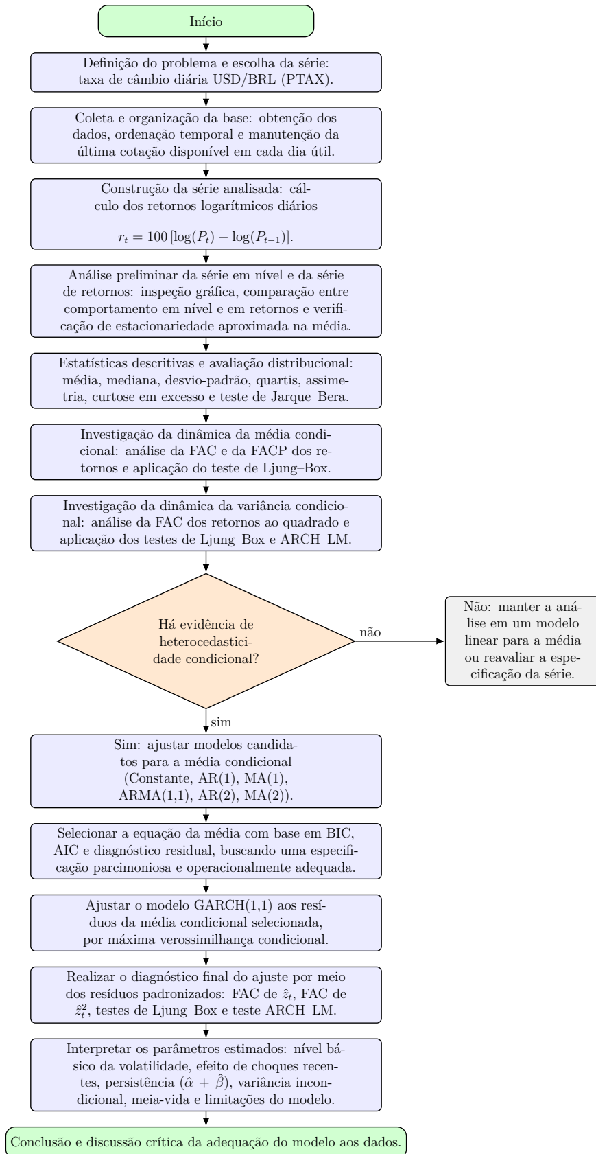
Figura 1: Fluxograma do método de análise adotado no trabalho.
