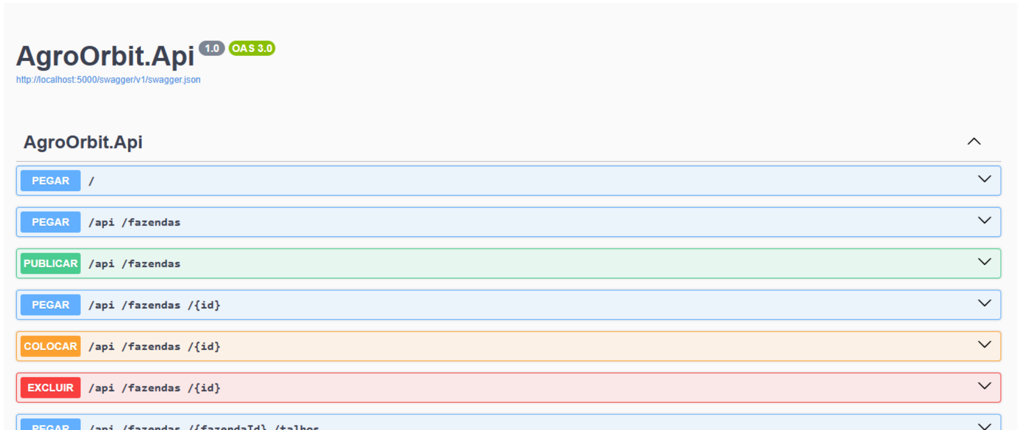
Figura - Swagger - endpoints de fazendas
