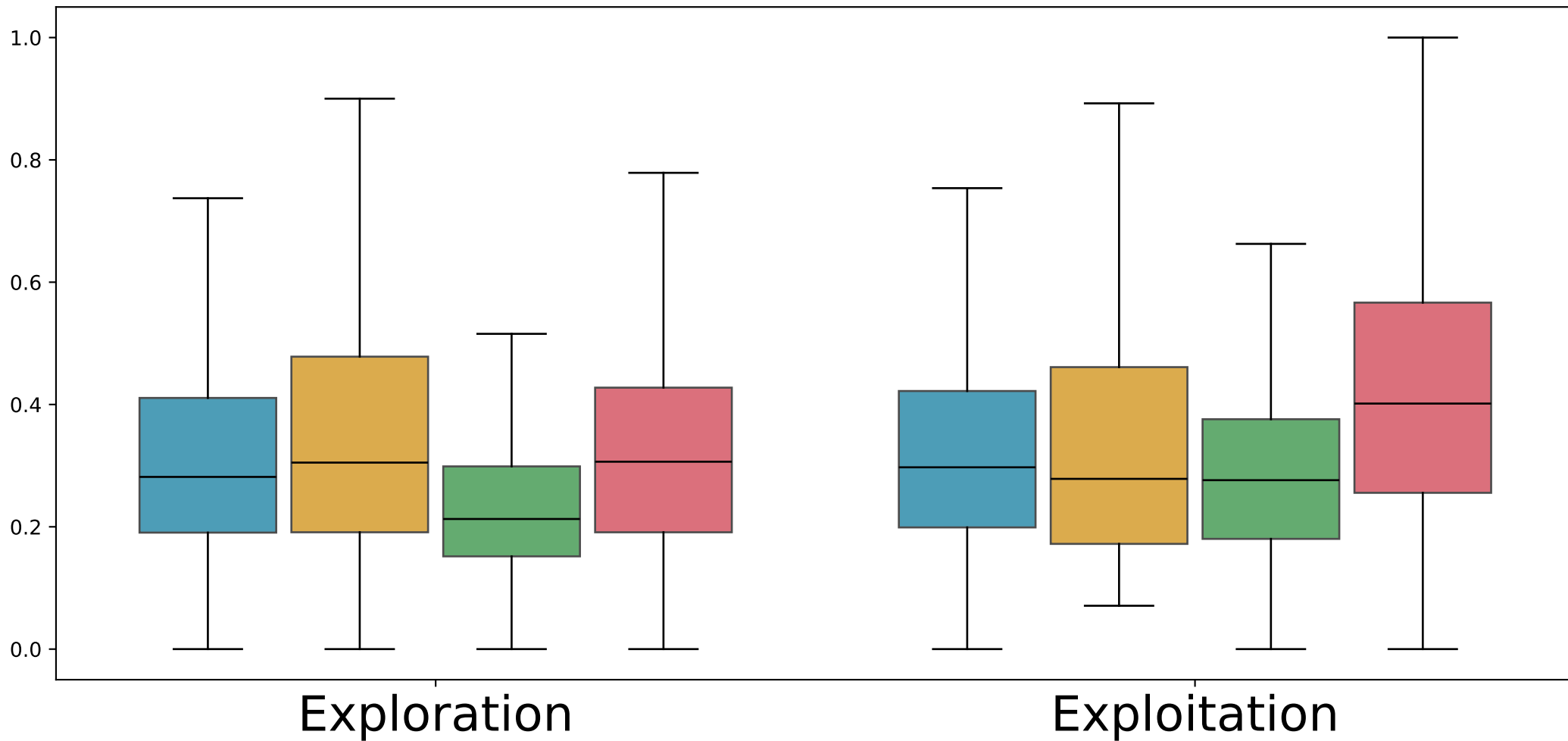
CodeBLEU Score
