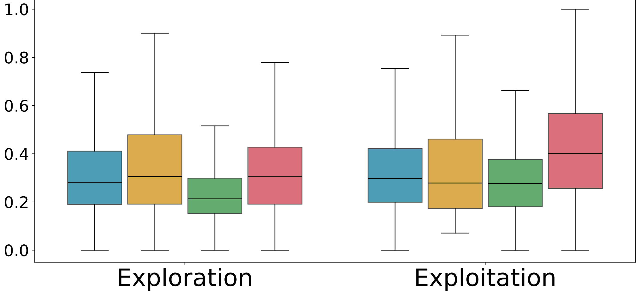
CodeBLEU Score
