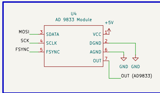
AD 9833 MODULE
