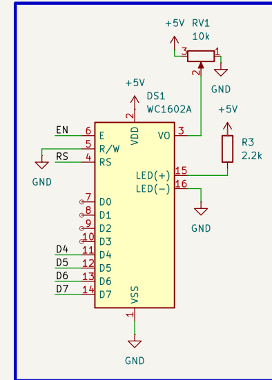
LCD 16x2
