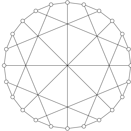
Slika 31: McGee graf je primer kletke, ki ni Mooreov graf. Je 3-regularen graf s premerom 4 in ožino 7.
