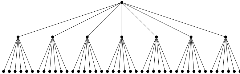
Slika 6: Mooreovo drevo T_{\Delta,D} je podgraf vsakega \Delta -regularnega Mooreovega grafa premera D . Na sliki je prikazan primer za \Delta = 7 in D = 2 .
