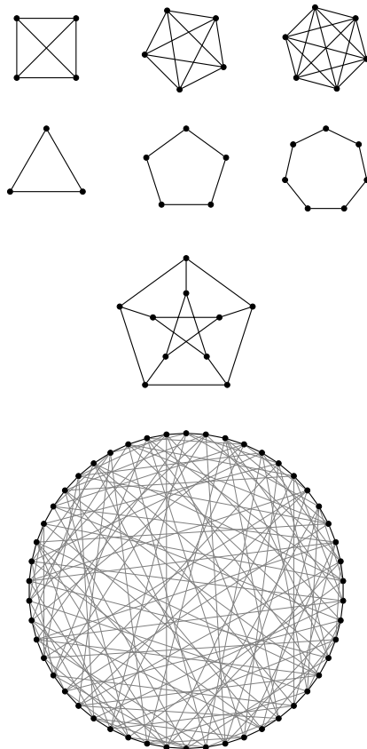
Slika 18: Obstajajo dve neskončni družini Mooreovih grafov in dva netrivialna grafa, medtem ko obstoj Aschbacherjevega grafa valence 57 ostaja odprto vprašanje.
