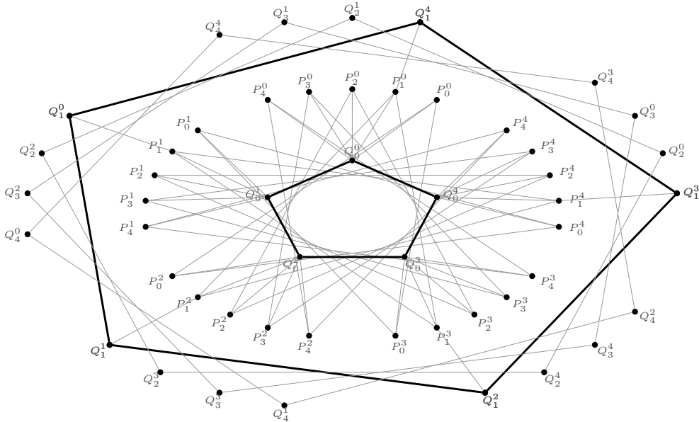
Slika 14: Podgraf Hoffman-Singletonovega grafa s centralnim ciklom Q_0 . Podgrafa \mathcal{H}_7[N_1(Q_0)] in \mathcal{H}_7[N_2(Q_0)] sta uniji disjunktne petkotnikov in petkotnikov.
