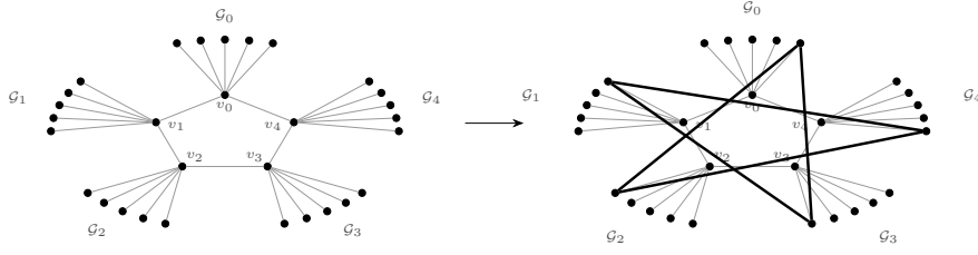
Slika 13: Petkotniki v podgrafu \mathcal{H}_7[N_1(Q) \cup Q] , napeti kot komplekturni petkotniki.
