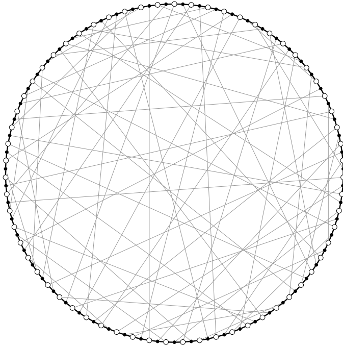
Slika 29: Incidenčni graf geometrije H(\text{GF}(2)) iz zgleda 3.61. Je 3-regularen dvodelni Mooreov graf ožine 12 in premera 6, znan tudi pod imenom Tutteova 12-kletka.
