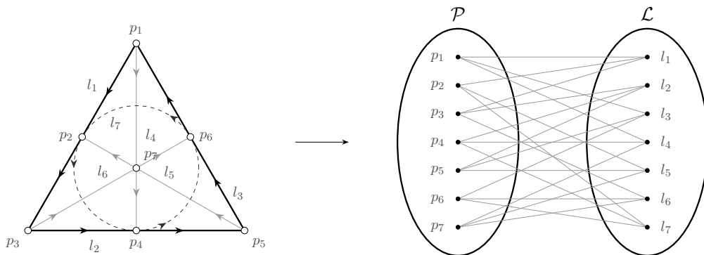
Slika 10: Fanova ravnina in njen incidenčni graf.
