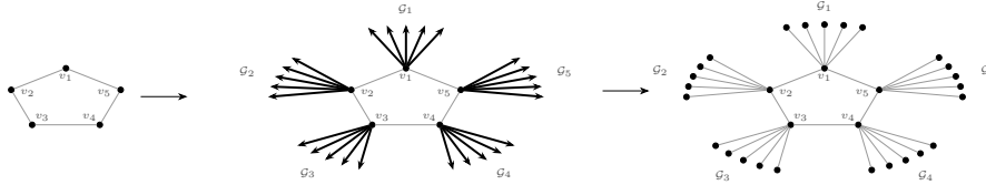
Slika 4: Centralni cikel in gručo v Hoffmann-Singletonovem grafu.
