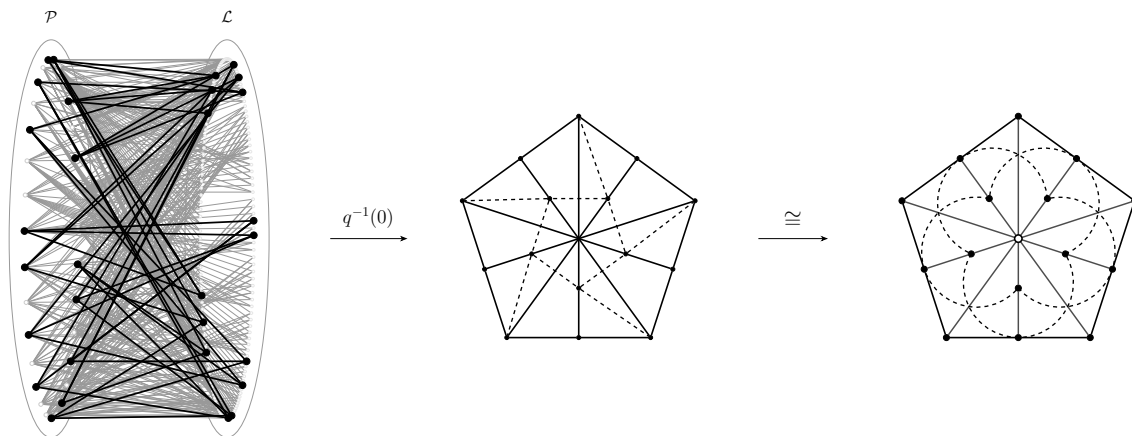
Slika 11: Posplošeni štirikotnik Q(4, \text{GF}(2)) \cong W(\text{GF}(2)) dobljen prek projektivnega prostora \text{PG}(4, \text{GF}(2)) s parabolično kvadratno formo q(x_0, x_1, x_2, x_3, x_4) = x_0x_1 + x_2x_3 + x_4^2 . Njegov incidenčni graf je 3-regulren graf ožine 8 in premera 4.
