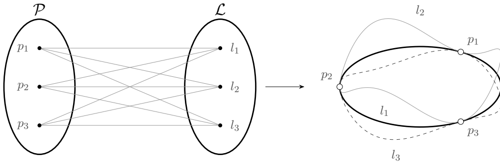
Slika 9: Posplošeni dvokotnik in njegov incidenčni graf.
