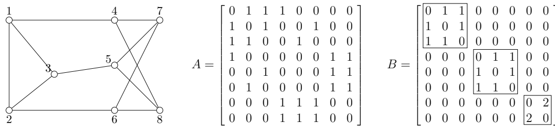
Slika 12: Graf (3, 2, -2) s pripadajočima matrikama (4.3).
