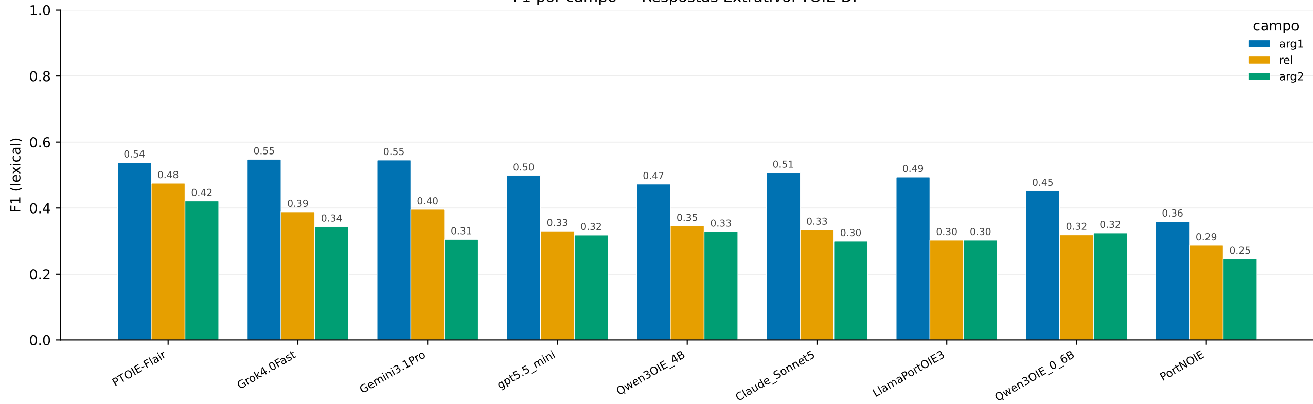
F1 por campo — Respostas ExtrativoPTOIE-DP
