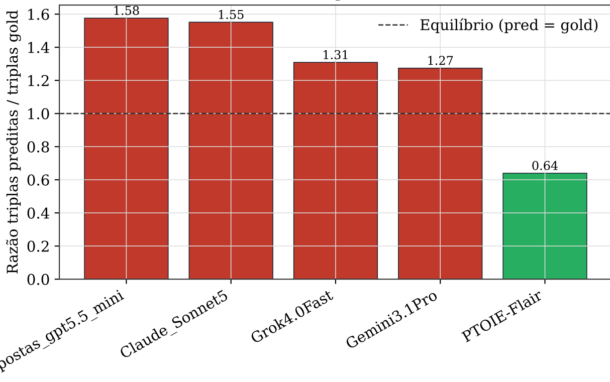
Razão Predito/Gold — Respostas ExtrativoPTOIE-DP
