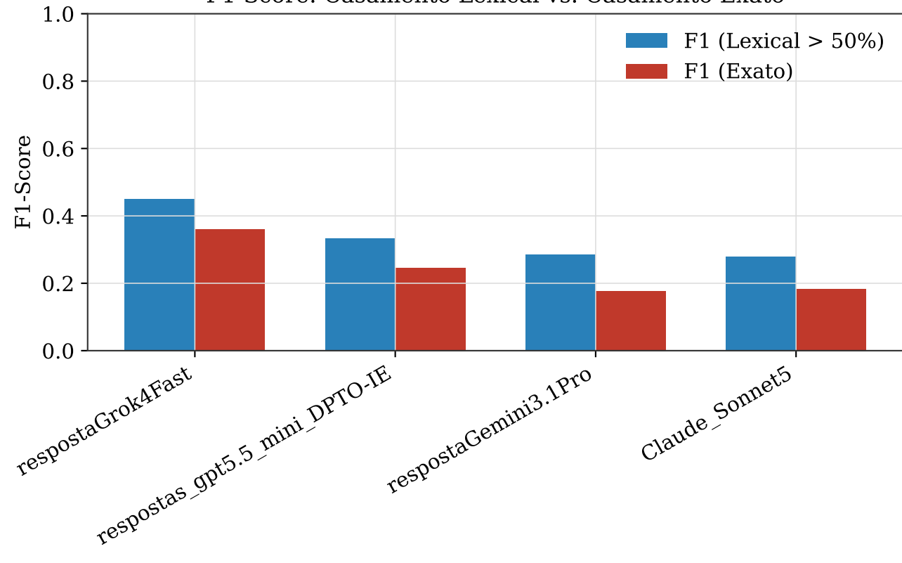
F1-Score: Casamento Lexical vs. Casamento Exato
