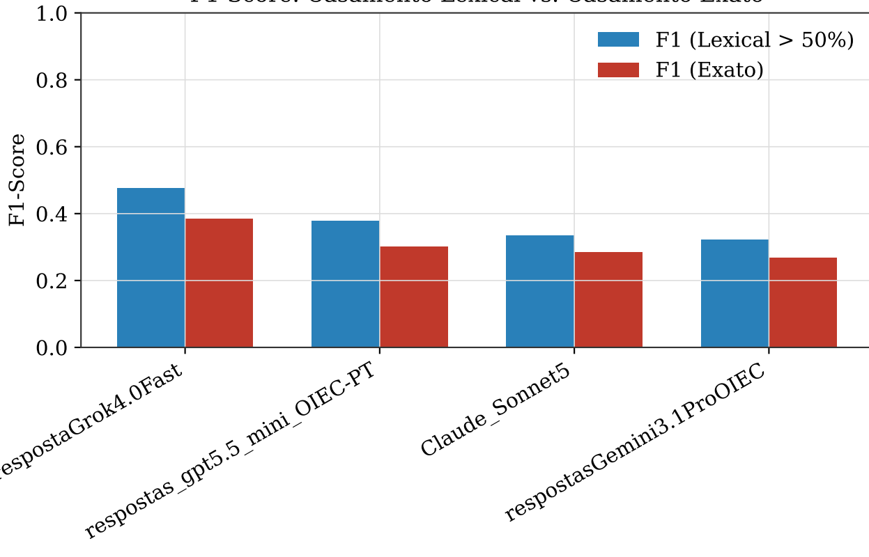
F1-Score: Casamento Lexical vs. Casamento Exato
