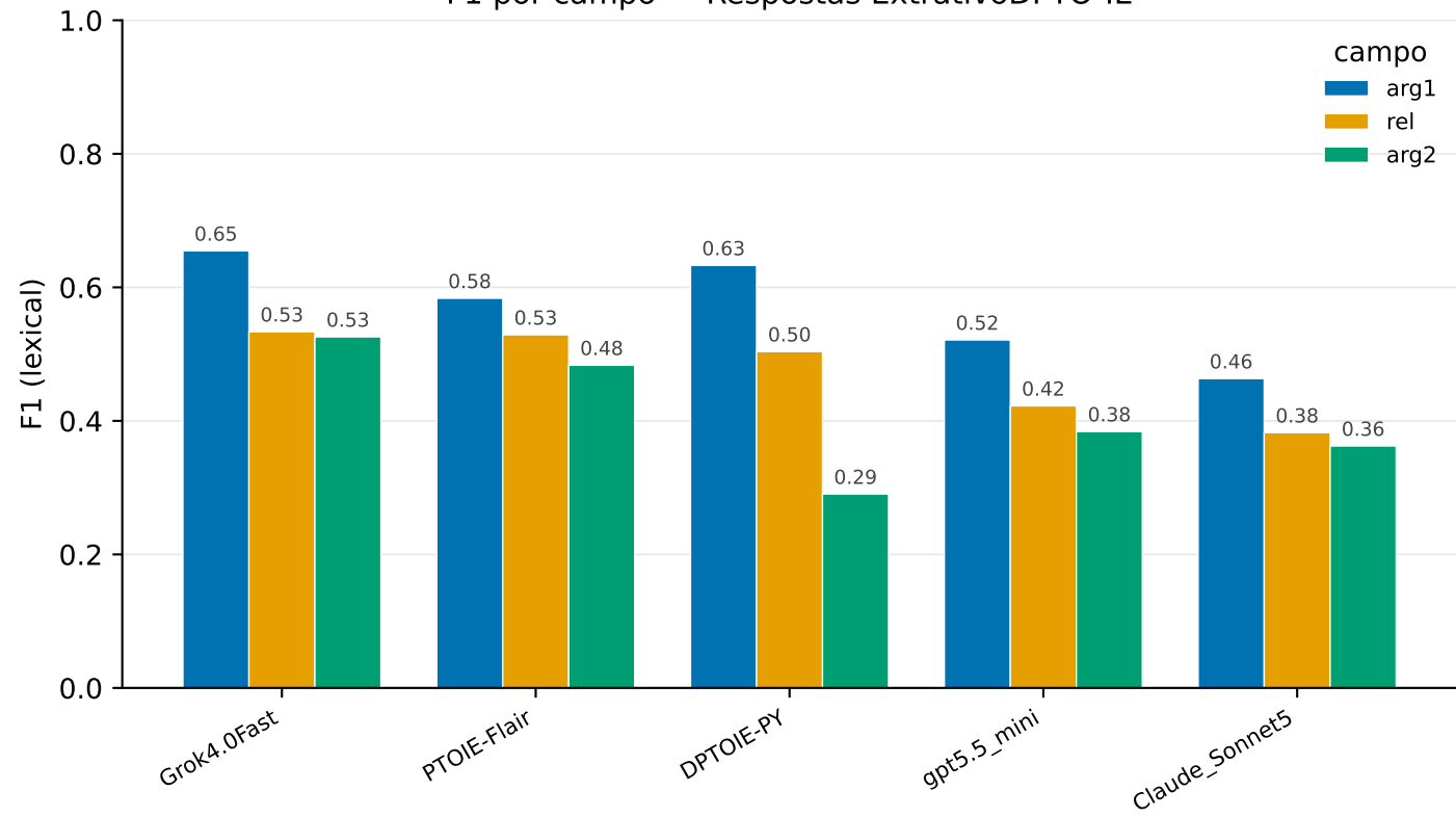
F1 por campo — Respostas ExtrativoDPTO-IE
