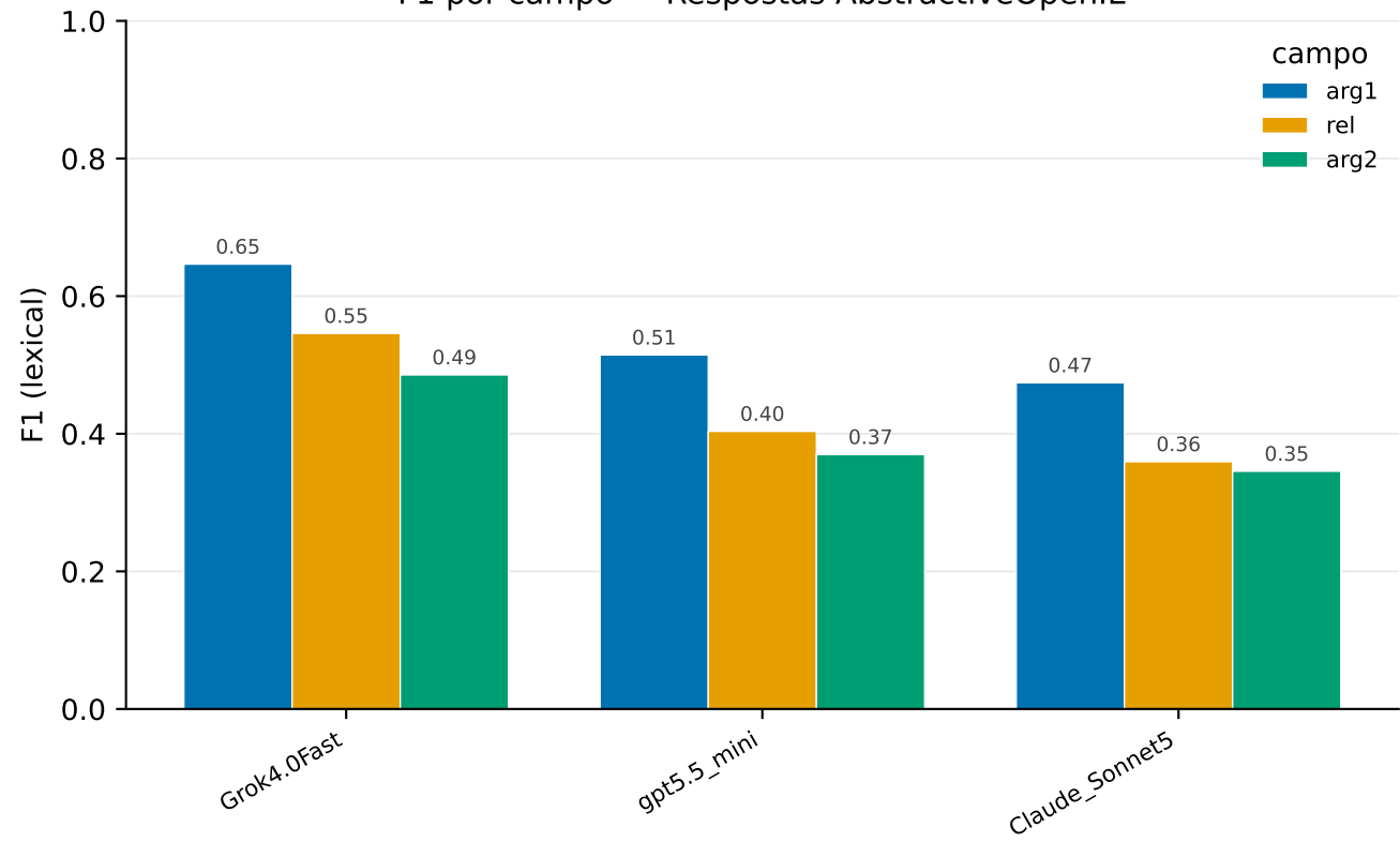
F1 por campo — Respostas AbstractiveOpenIE
