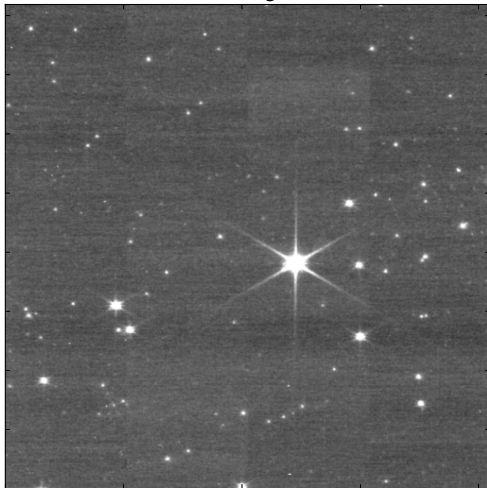
Im2 : Background
