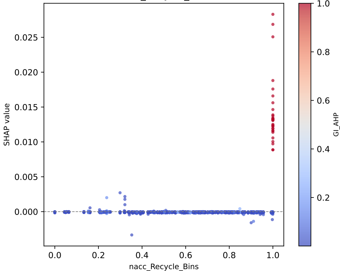
nacc_Recycle_Bins
