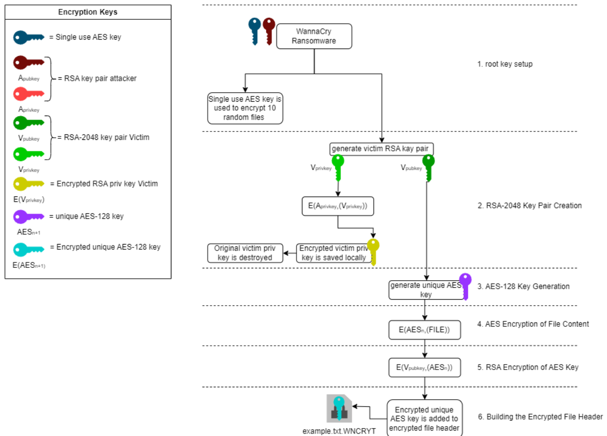
figuur 12 Encryptie proces diagram
