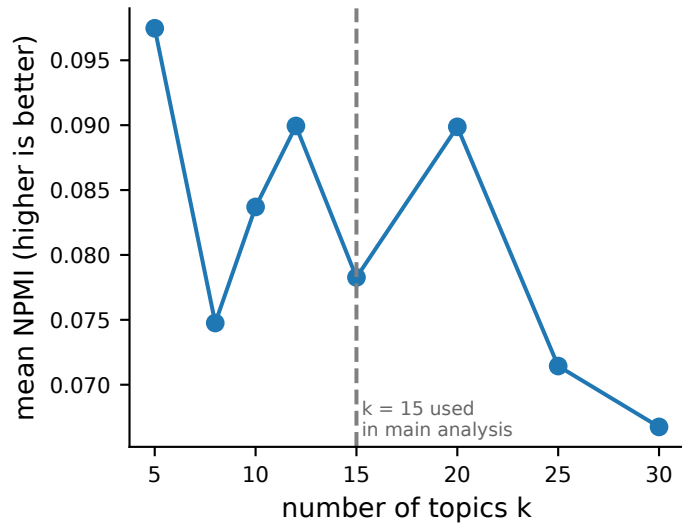
NPMI coherence
