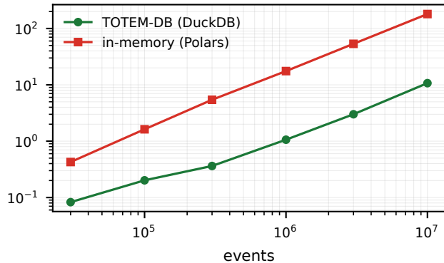
TOTeM discovery
