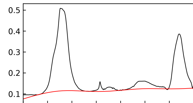
Ih 113 K
