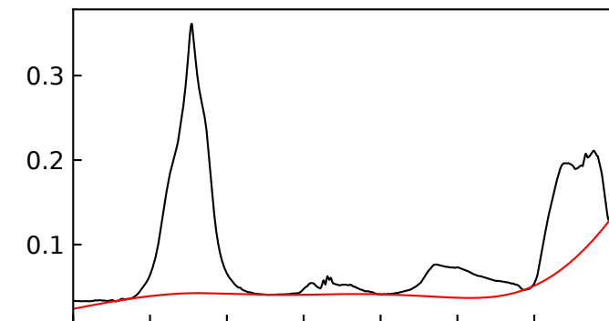
IceV 143 K
