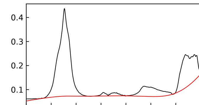
IceV 168 K
