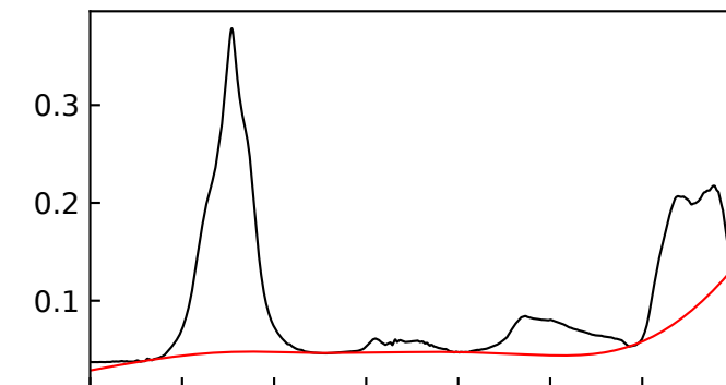
IceV 148 K
