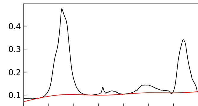
IceV 188 K
