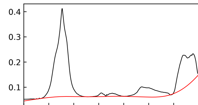
IceV 158 K
