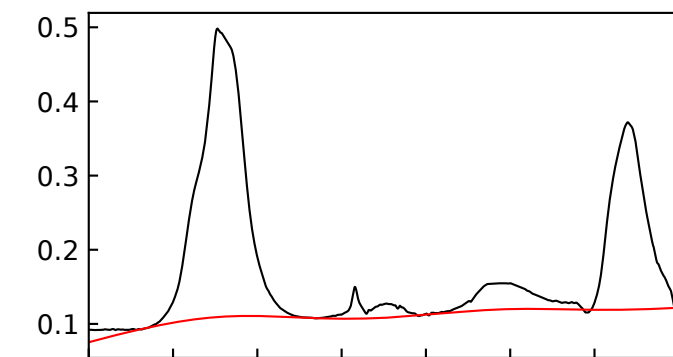
Ih 108 K
