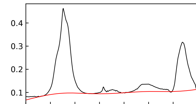
IceV 183 K
