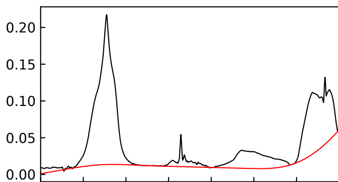
IceV 128 K
