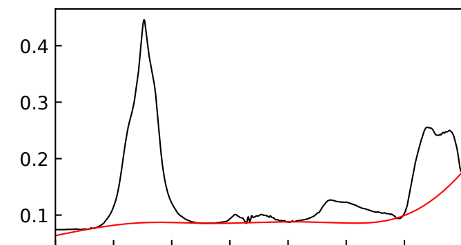
IceV 173 K
