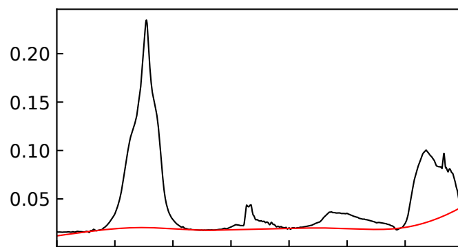
IceV 133 K
