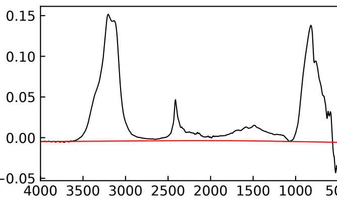
Ih 113 K
