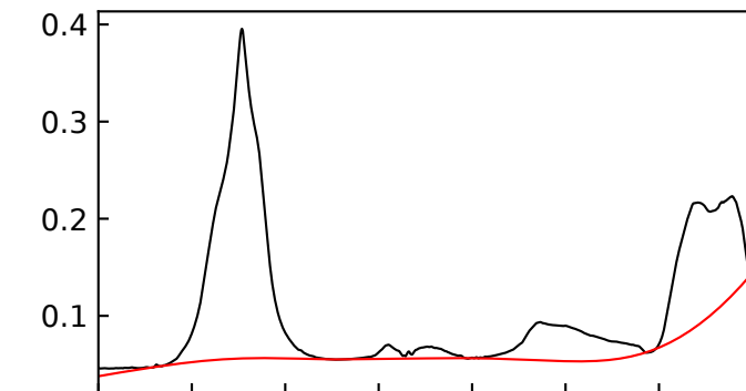
IceV 153 K
