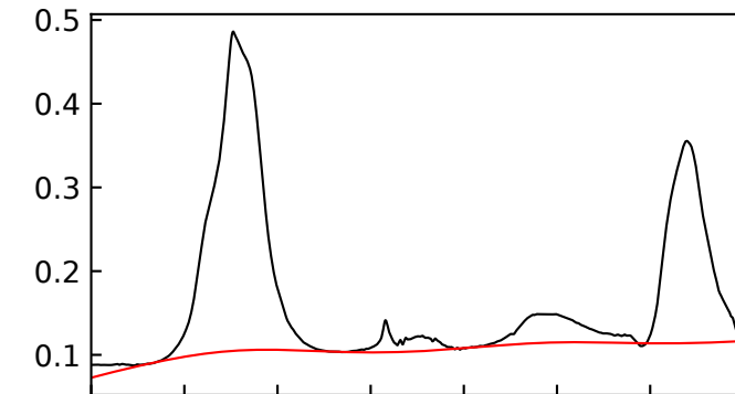
IceV 193 K
