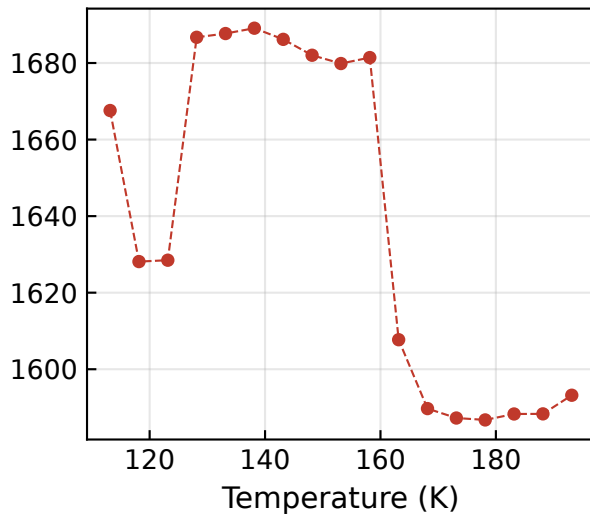
Bending ( 1800\text{--}1200\text{ cm}^{-1} )
