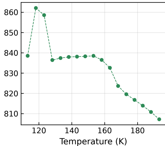
Libration ( 1000\text{--}550\text{ cm}^{-1} )
