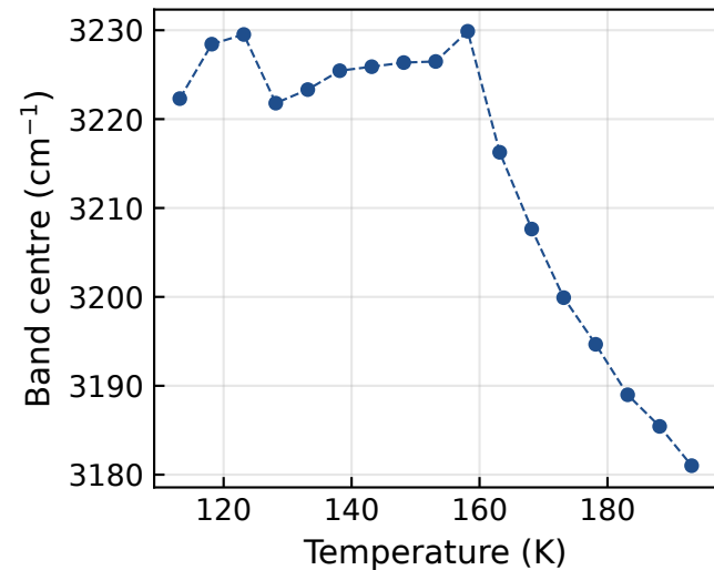
Stretching ( 3500\text{--}3000\text{ cm}^{-1} )
