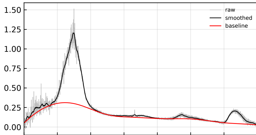
ice Ih: IceIh_100K
