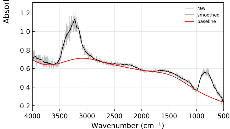
ice Ih: IceIh_100K
