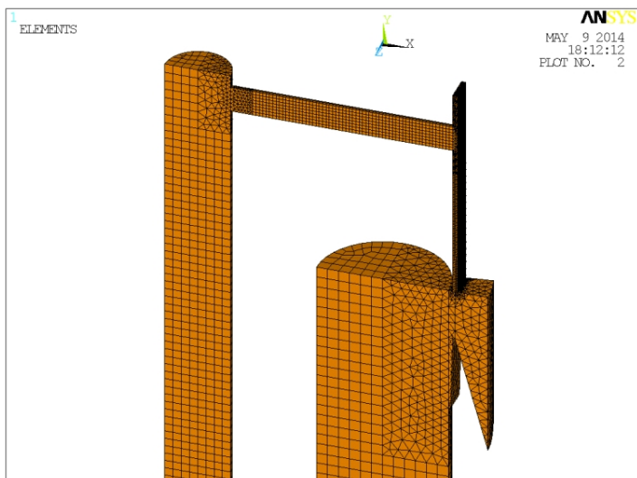
Figure 5: Obrázok z ANSYS-u.
