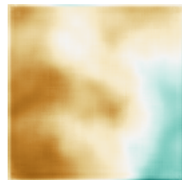
DEM
