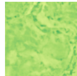
NDVI
