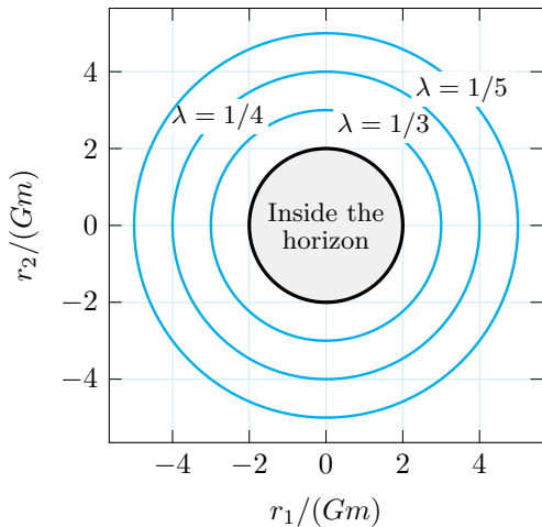
Schwarzschild: spatial contours
