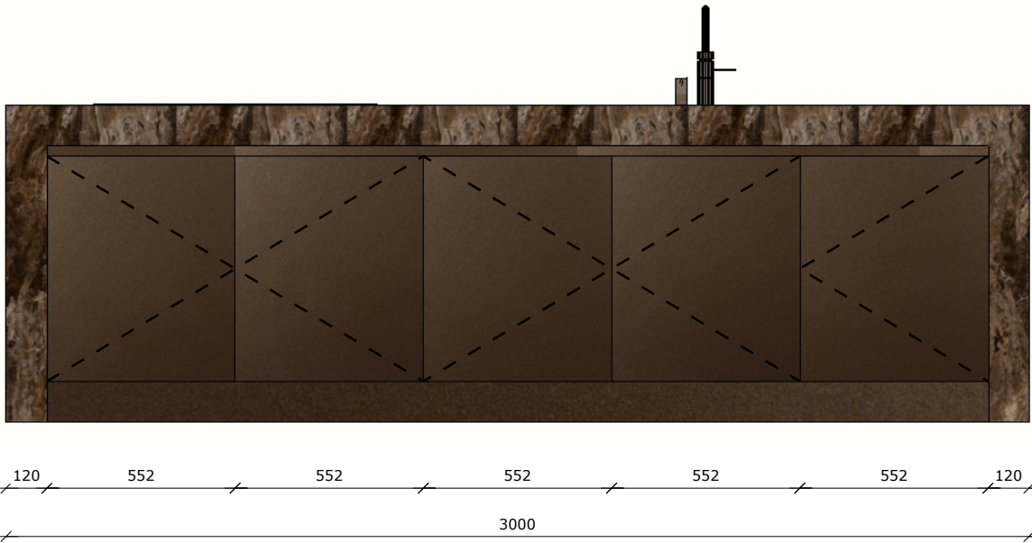
VOORAANZICHT
