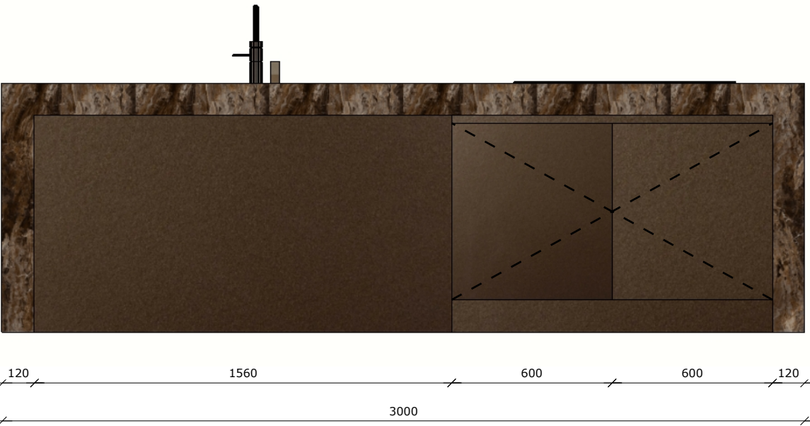
ACHTERAANZICHT
