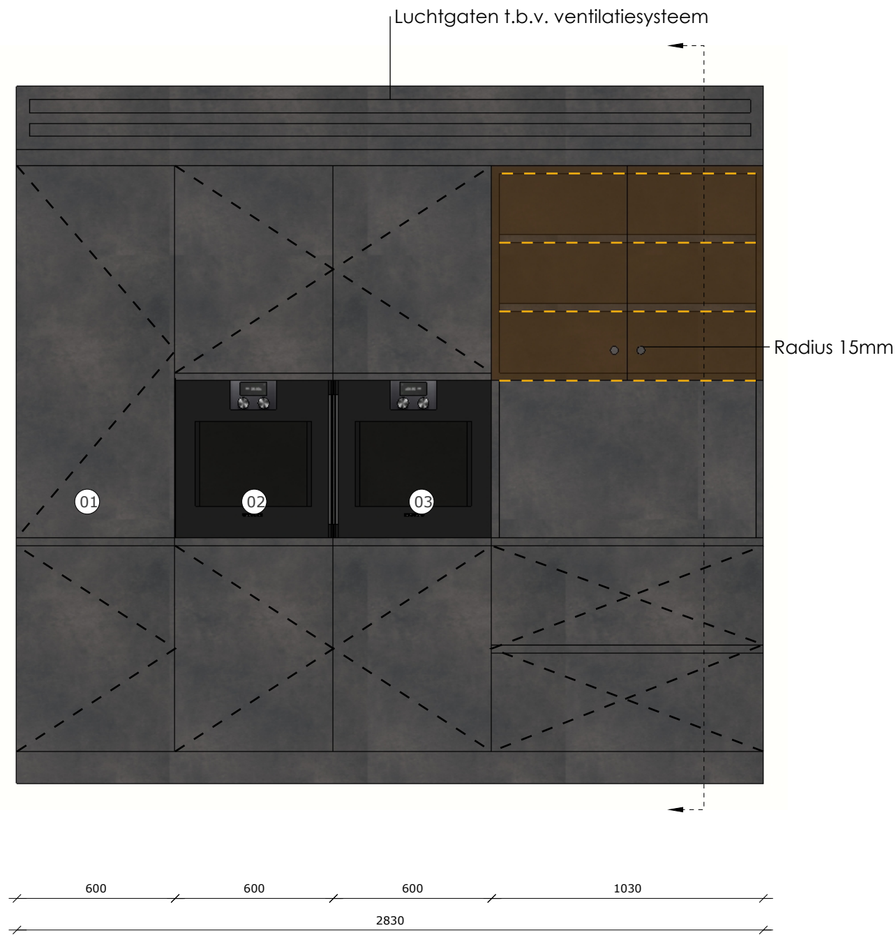
VOORAANZICHT
