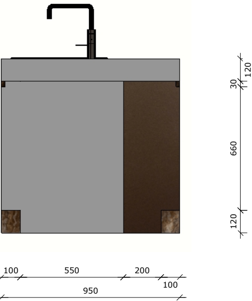
DOORSNEDE
