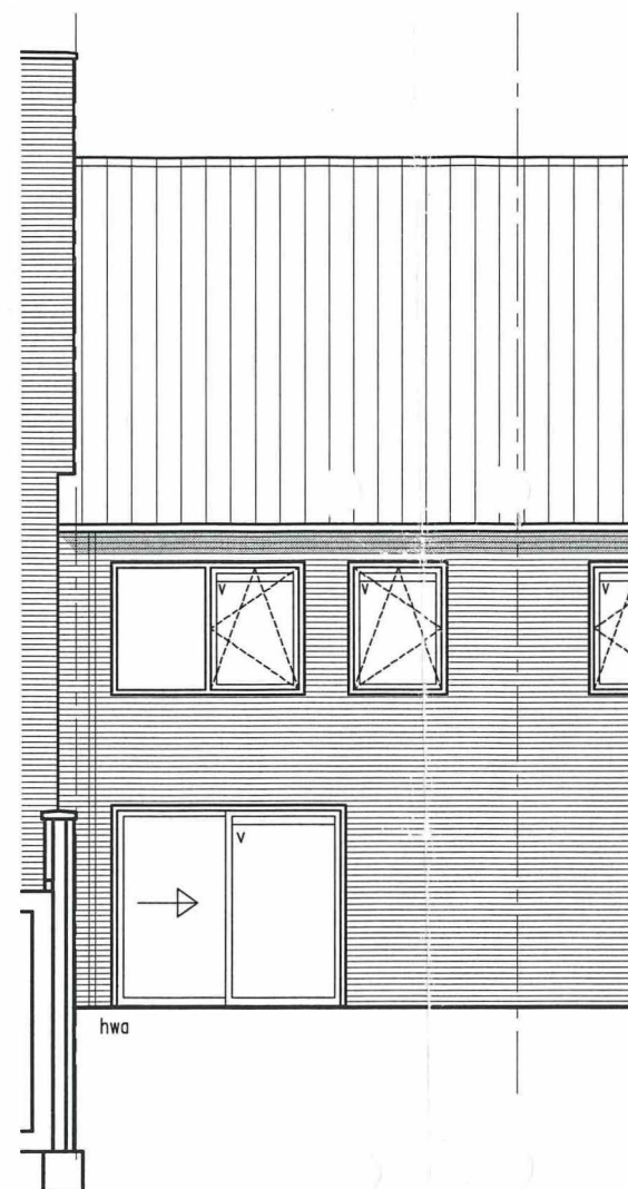
achtergevel
