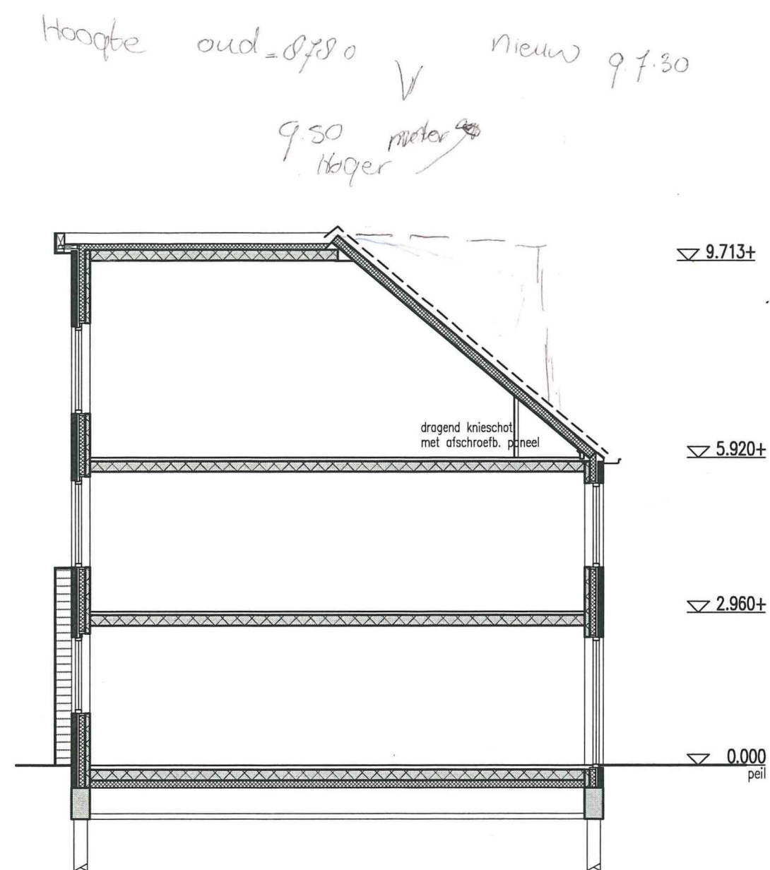
doorsnede
