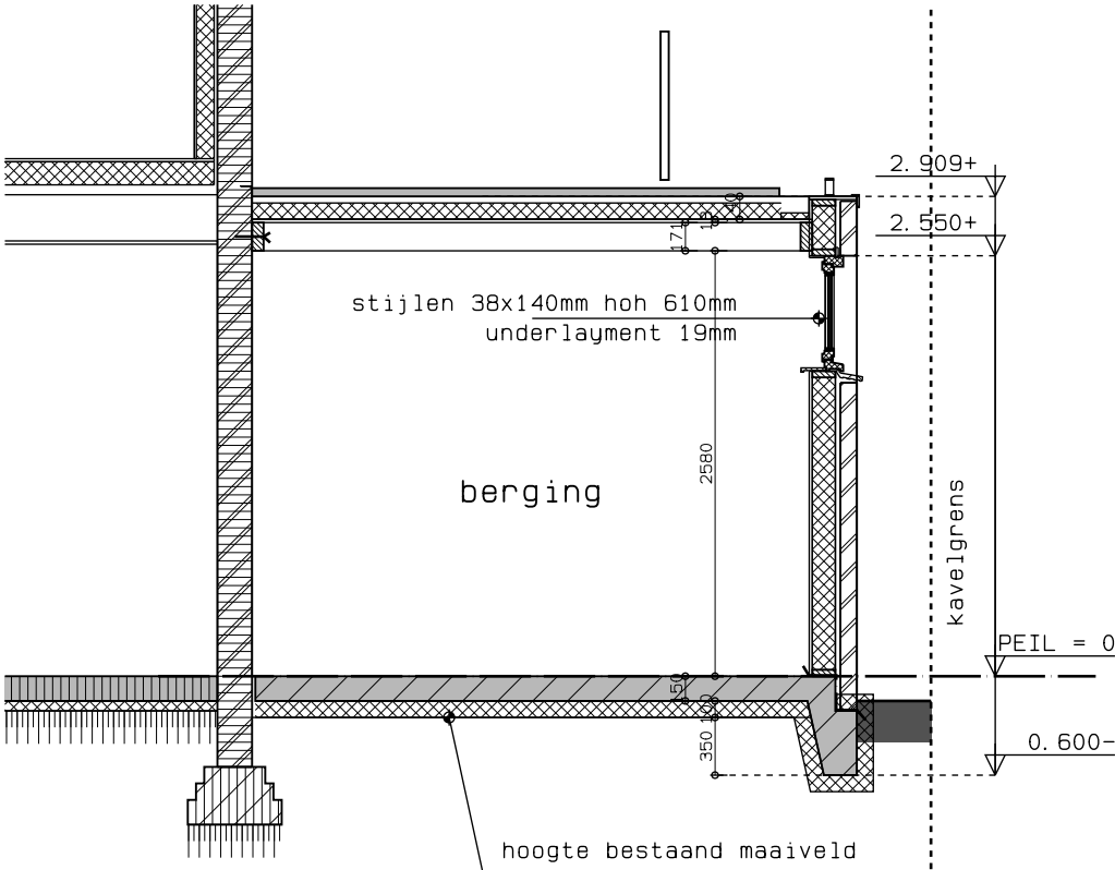
doorsnede C-C
