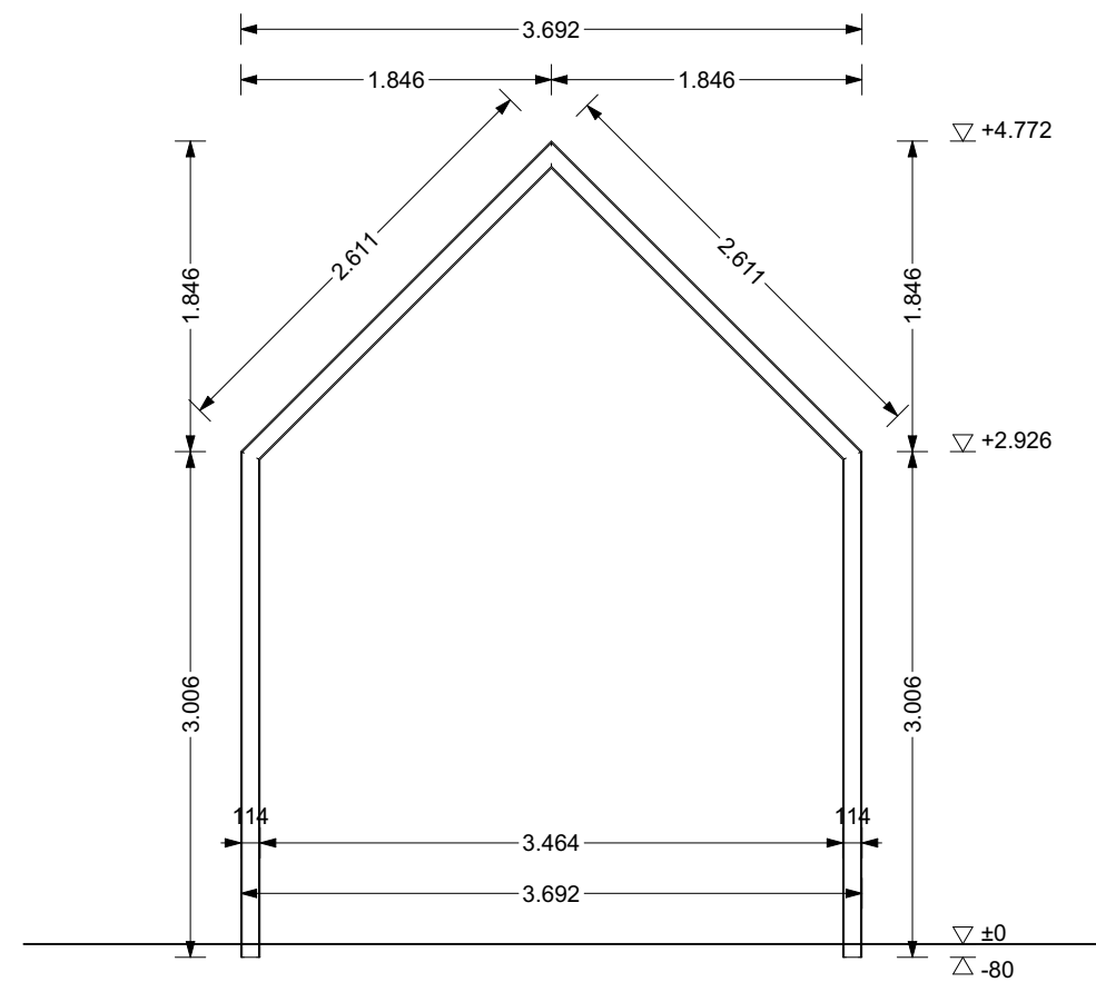
stalen spantconstructie
