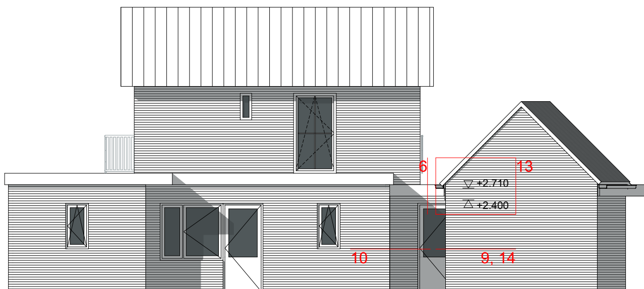
achtergevel
