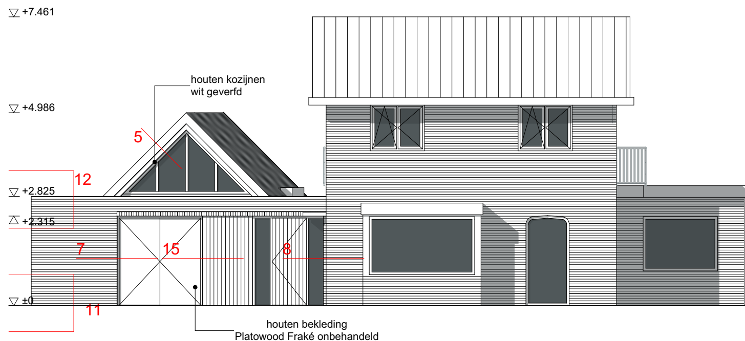
voorgevel
