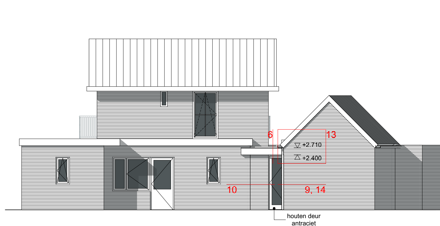
achtergevel
