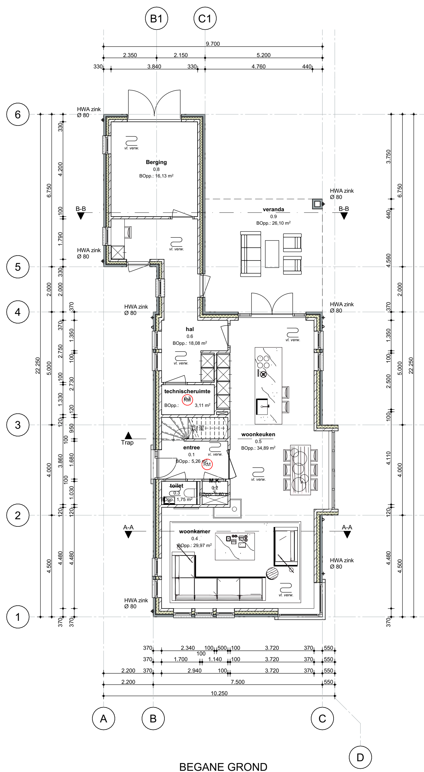
BEGANE GROND
