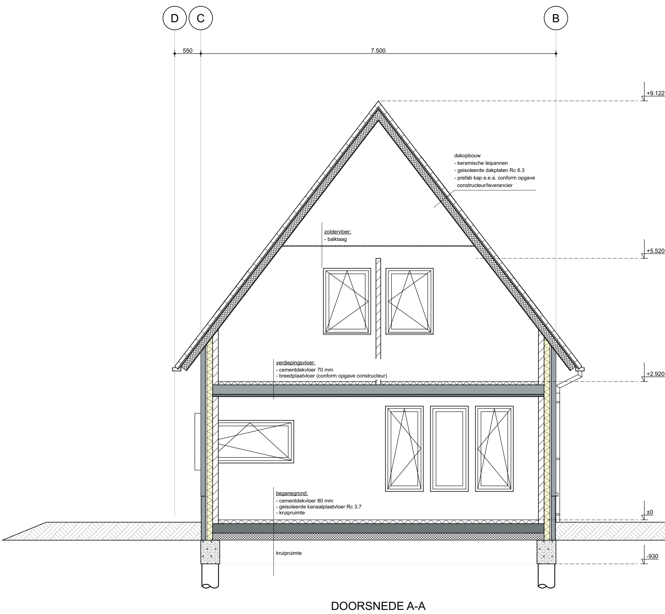
DOORSNEDE A-A
