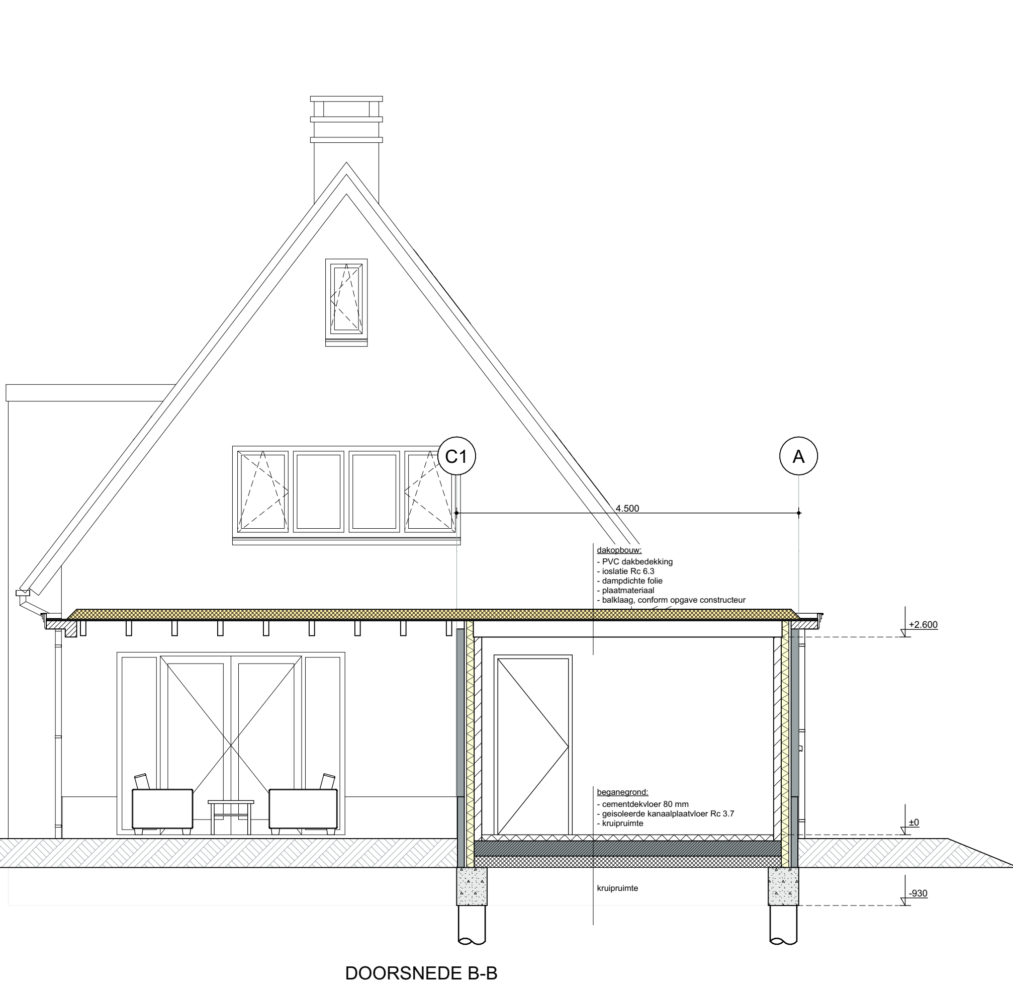
DOORSNEDE B-B
