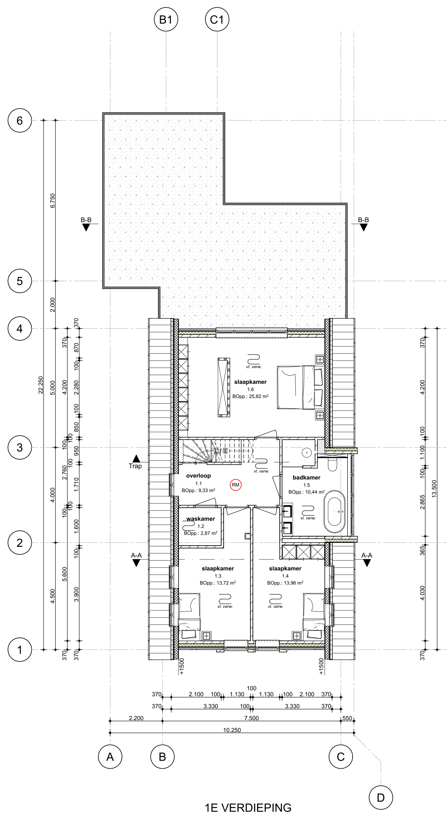
1E VERDIEPING
