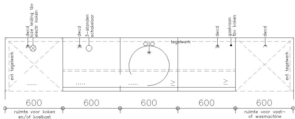
Bovenaanzicht
