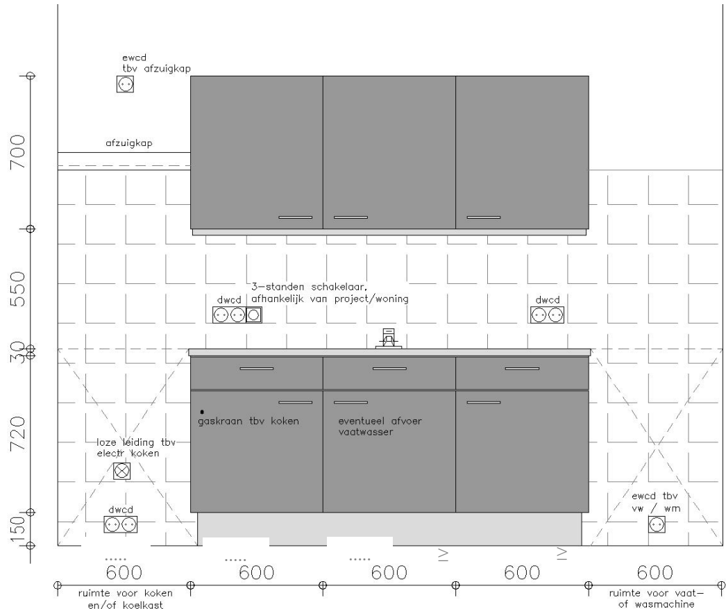
Vooraanzicht
