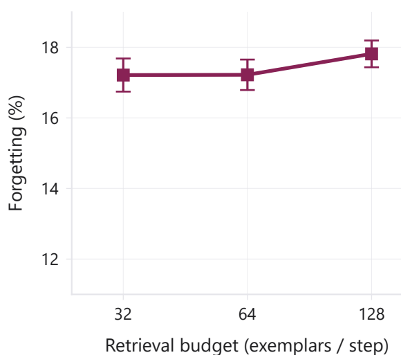
(d) Retrieval budget — Forgetting
